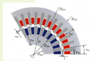
Modélisation mécanique
