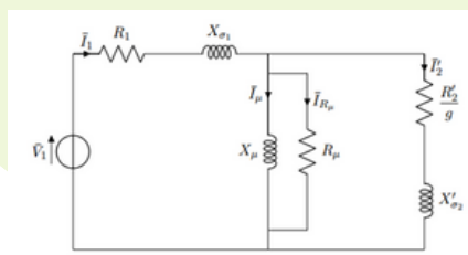
Modélisation électrique
