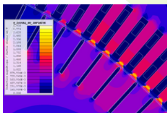
Modélisation thermique
