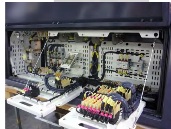
Distribution électrique de train
